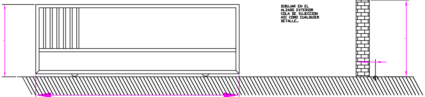
ALZADO VISTA EXTERIOR
